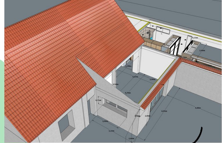
Région de FRUGES : Projet d'extension d'une maison (phase esquisse)
